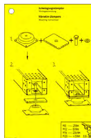
61715 – Amortisseur de vibration
