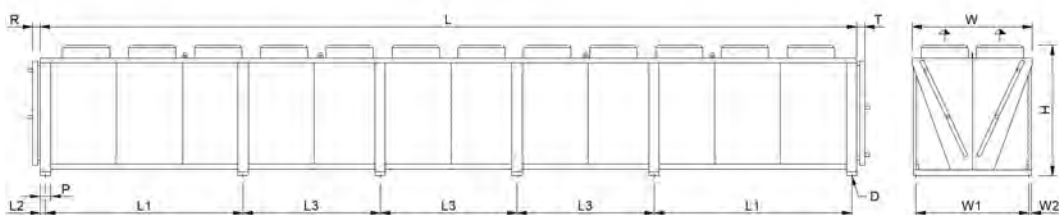
Cotations (raccords des deux côtés)
