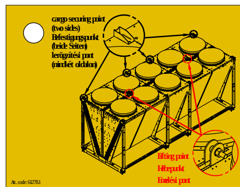
61278.1 – Point de levage et de fixation
