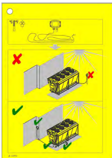
69793 – Installation de capteur de température (pour hydro-BLU™)
