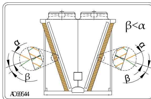
69544 – Installation d'un média humidifié (pour hydro-BLU™)
