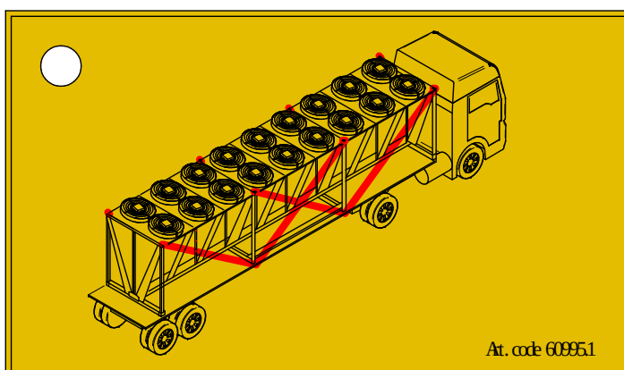
60995.1 – Anneau d'arrimage
