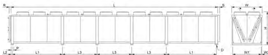
Cotations (raccords d'un côté)
