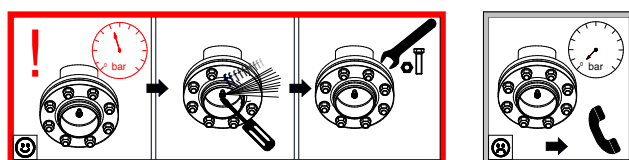
70722 – Remplissage de la pression de transport
