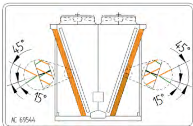
69544 - Installation d'un média humidifié (avec hydroBLU)
