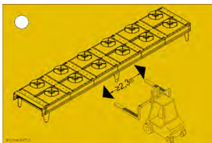
61072.1 – Plage d'utilisation pour chariot de manutention à fourche pour appareils à deux rangées
