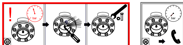
70722 – Remplissage de la pression de transport
