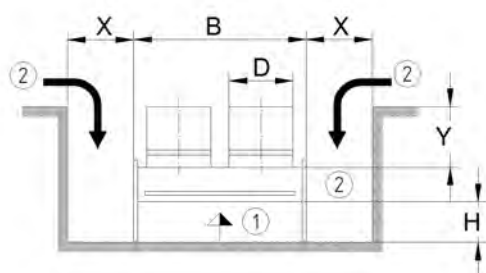
Installation dans un renforcement – buses de sortie d'air
