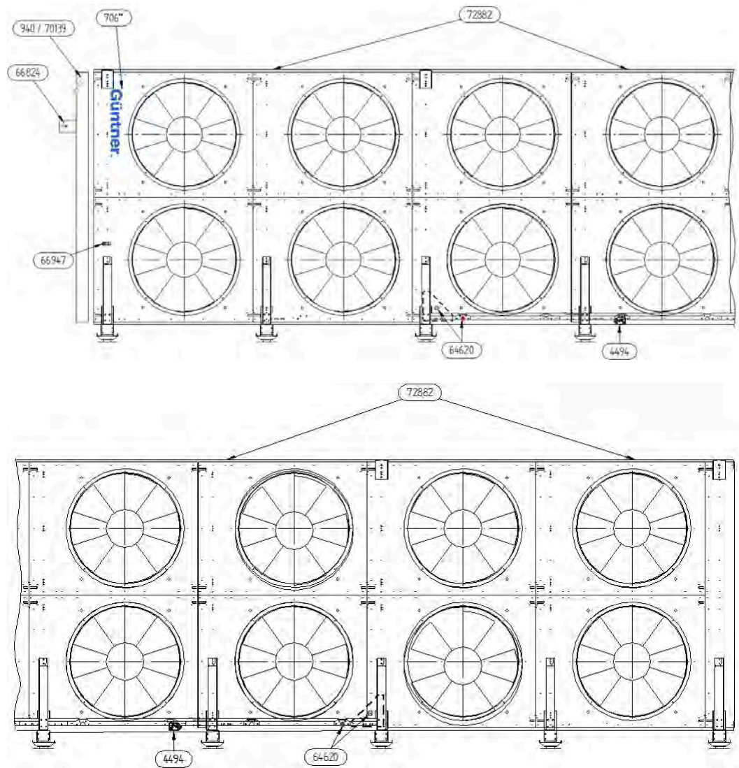
Vues du type II
