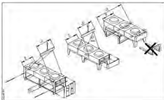
Illustration des opérations de transport pour FLAT VARIO
