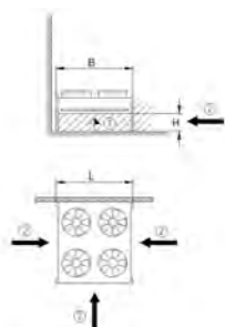
Installation contre un mur de bâtiment
