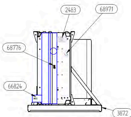
Vues du type I
