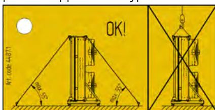
5828.1 – Emploi d'une grue ou d'un chariot de manutention à fourche pour les appareils de type II + III
