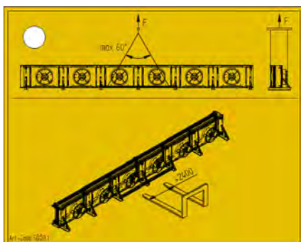
61072.1 – Plage d'utilisation pour chariot de manutention à fourche pour appareils à deux rangées
