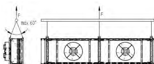
Illustration des opérations de transport pour Vertical VARIO de type I
