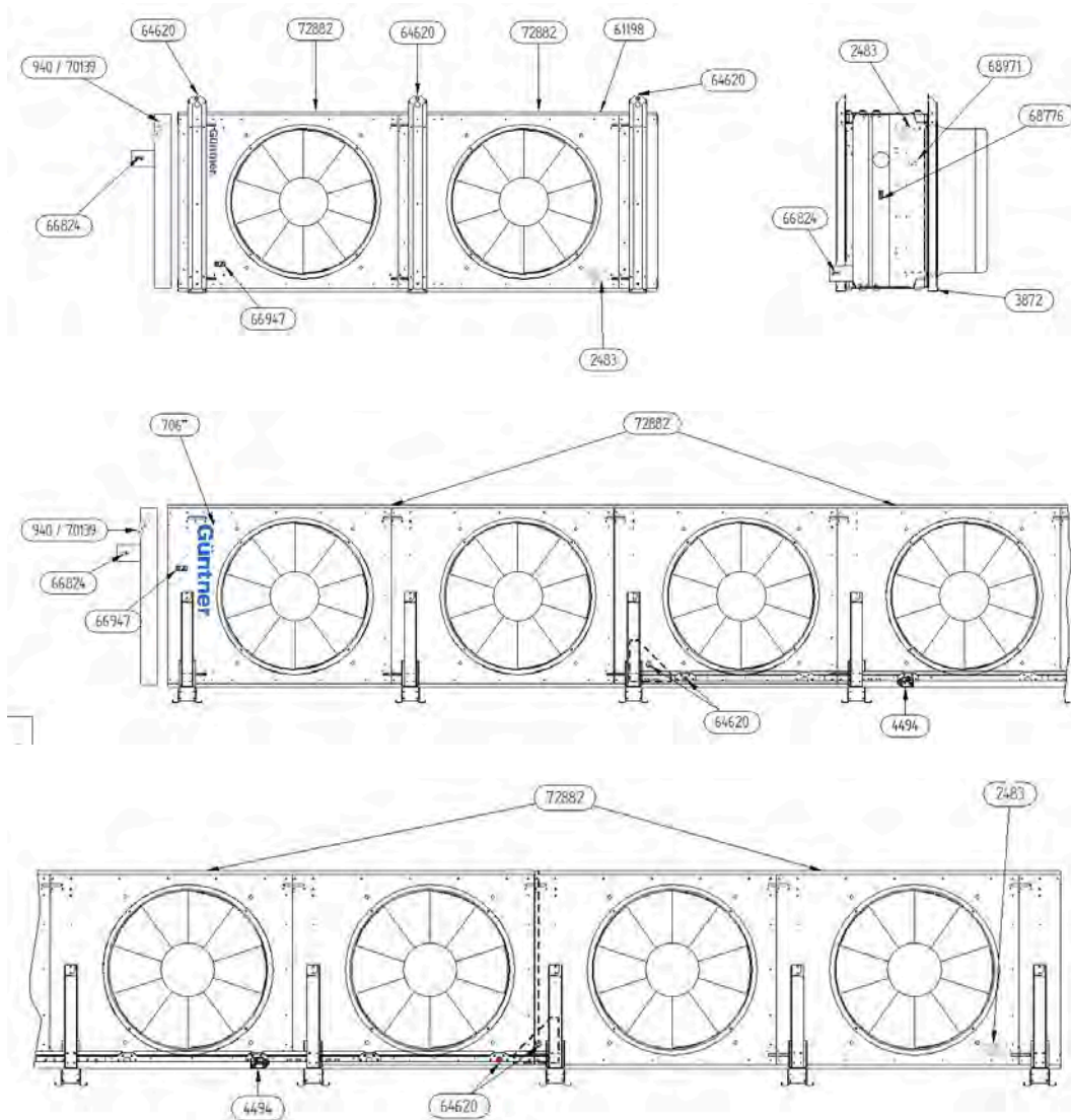
Vues du type I
