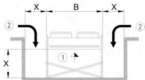
Installation dans un renforcement
