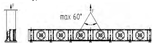
Illustration des opérations de transport pour Vertical VARIO de types II+ III
