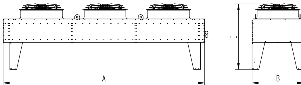
Exemple du type GCHV
