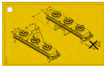
3631.1 – Règle de transport pour appareils Flat
