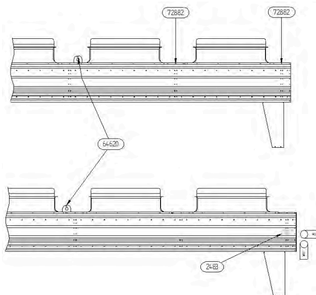
Vues séparées A (en haut) et B (en bas) – côté droit
