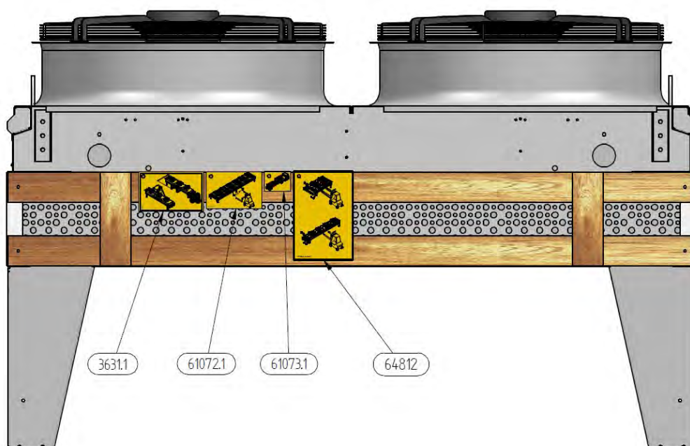
Verpackung Flat
