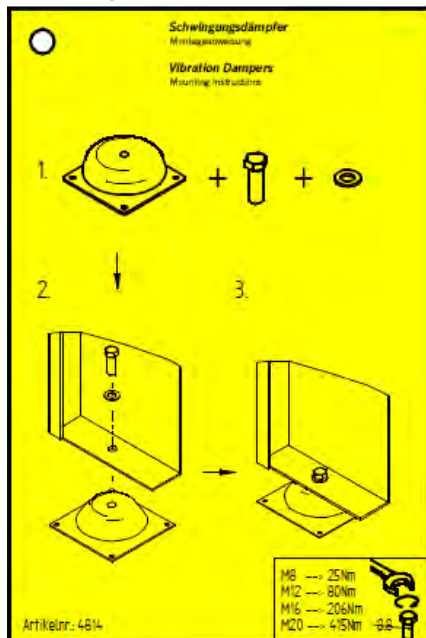
4814 – Hinweis zu Schwingungsdämpfern (für Typ I)
