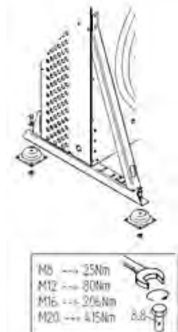
Darstellung des Transportprinzips beim Vertical VARIO Typen II und III
