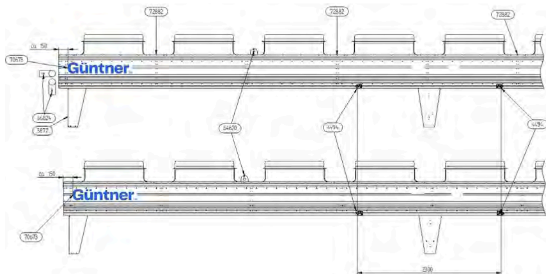
Geteilte Ansichten A (oben) und B (unten) – linke Seite
