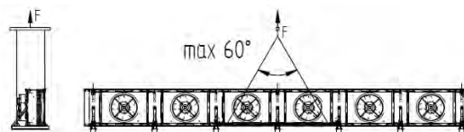
Darstellung des Transportprinzips beim Vertical VARIO Typen II und III
