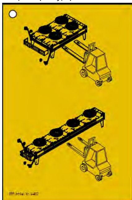
64812 – Entpackung Verflüssiger/Rückkühler
