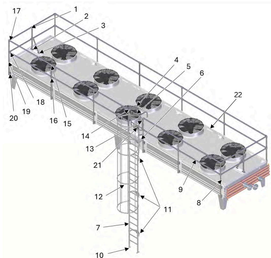
Einreihige Absturzsicherung
