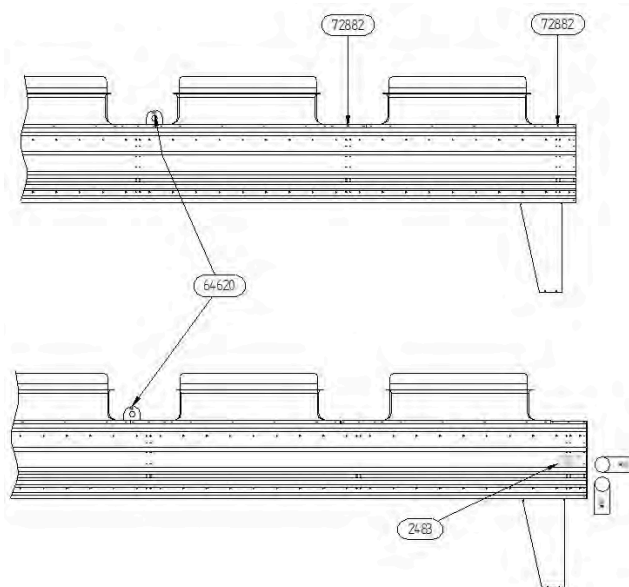
Geteilte Ansichten A (oben) und B (unten) – rechte Seite
