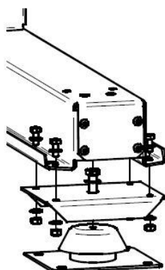
Typ II und III
