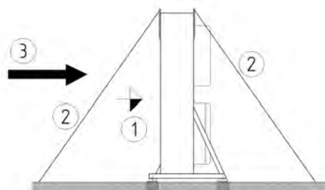
Freie Montage
