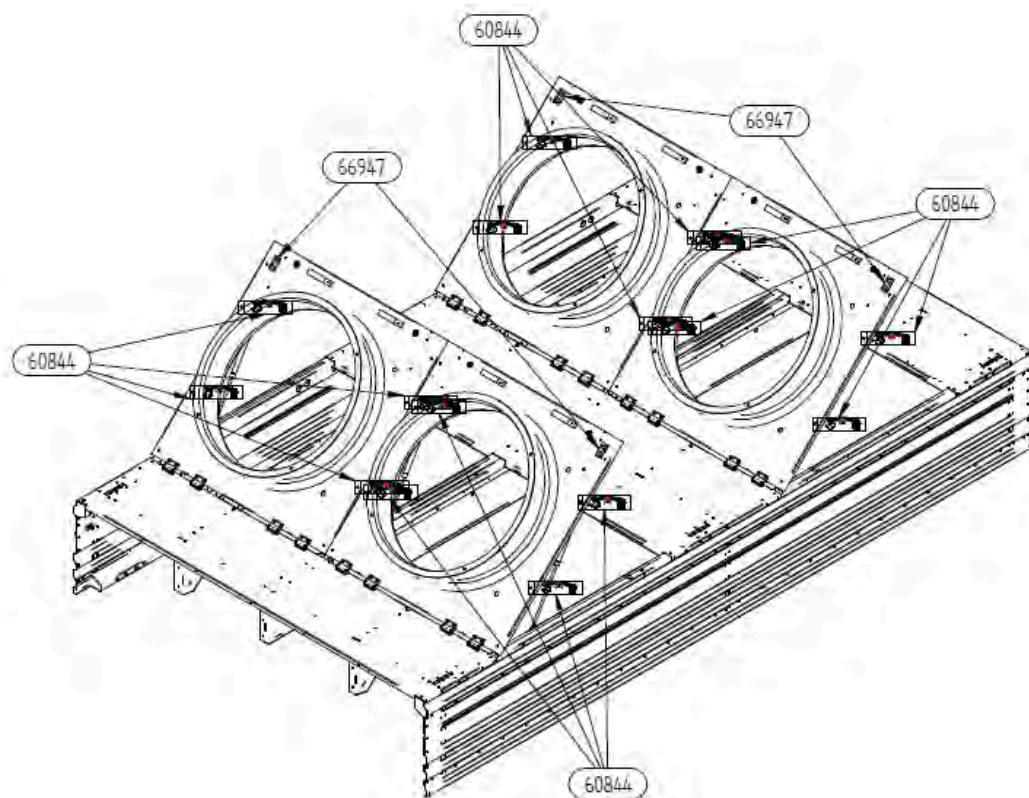
Ansicht bei klappbaren Ventilatorplatten (Zubehör)
