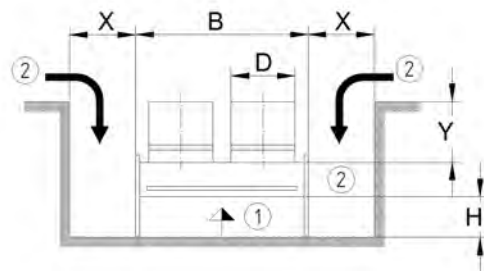
Montage in einer Vertiefung – Ausblasdüsen
