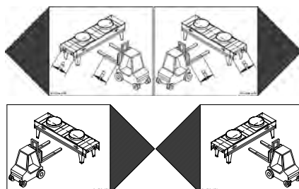
4494 – Einsatzbereich für Flurförderzeuge mit Gabeln mit Positionspfeilen
