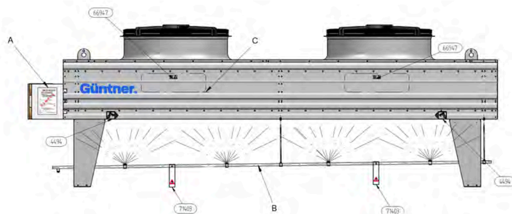
Platzierung von Kennzeichnungen auf dem Gerät (mit optionalem Wassersprühsystem)
