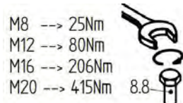
Typ II und III
