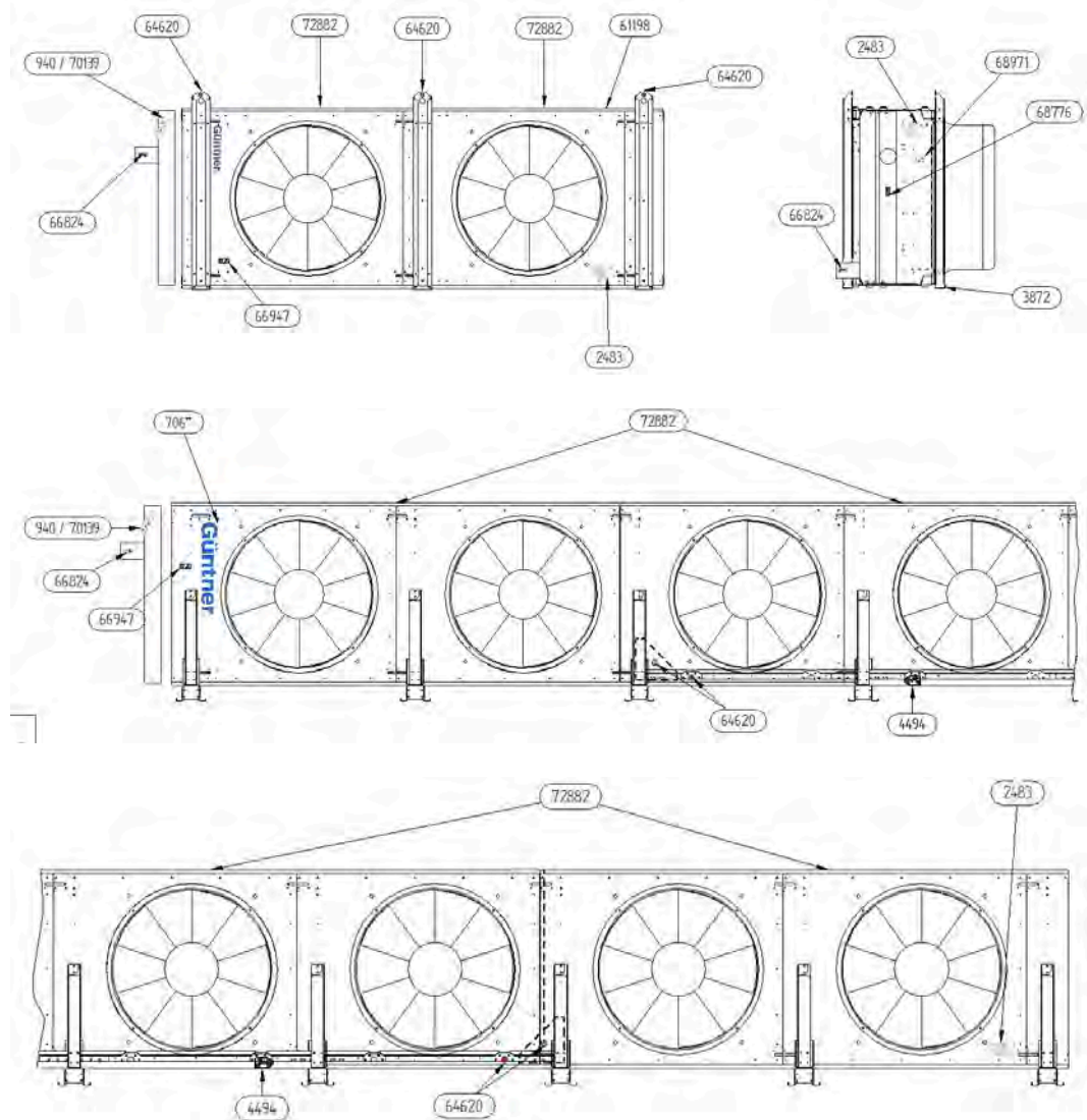
Ansichten Typ I
