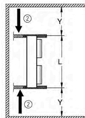
Wandmontage; Seitenansicht (oben) und Ansicht von oben (unten)
