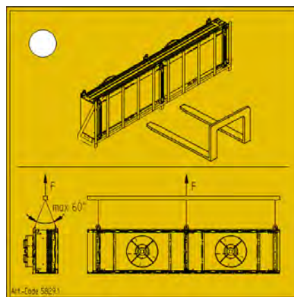
5829.1 – Einsatz eines Krans oder Flurförderzeugs mit Gabeln für Geräte Typ I
