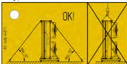
5828.1 – Einsatz eines Krans oder Flurförderzeugs mit Gabeln für Geräte Typ II + III
