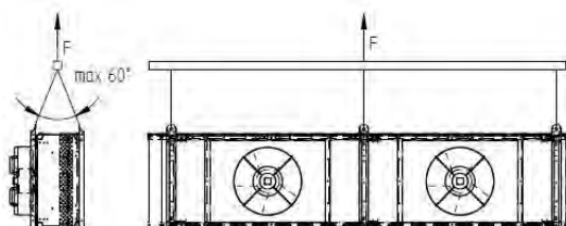
Darstellung des Transportprinzips beim Vertical
