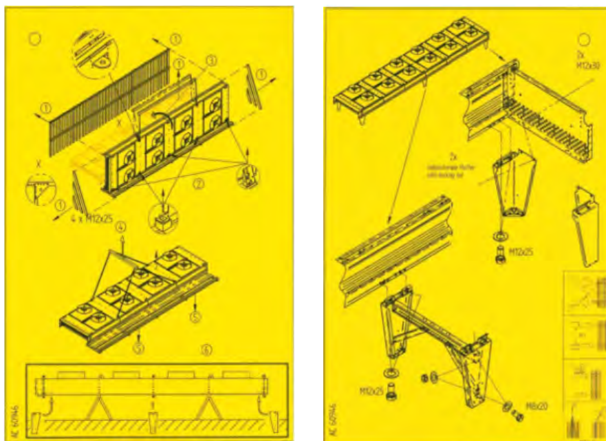
60946 – Entfernen der Palette und Aufbau des Geräts
