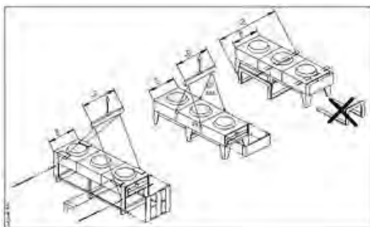
Darstellung des Transportprinzips beim Flat VARIO
