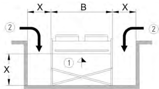
Montage in einer Vertiefung
