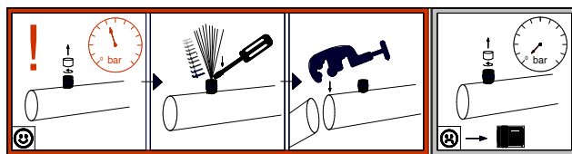
940 – Transportfüllung am Schraderventil
