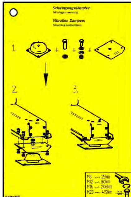
4492 – Hinweis zu Schwingungsdämpfern (für Typ II und III)
