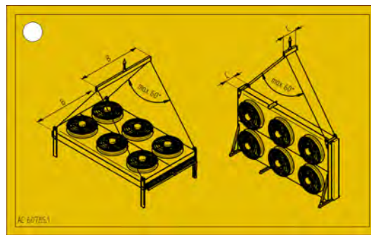
60785.1 – Règle en matière de transport (modules B, C et D)
