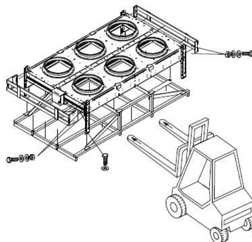
Déballage d'appareils horizontaux
