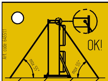
64551.1 – Remarque concernant le haubanage (modules B, C et D)
