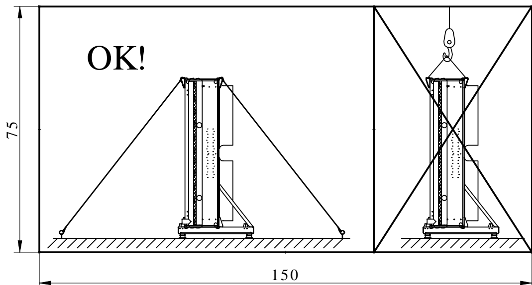
Tensionare curea conform SP 08
