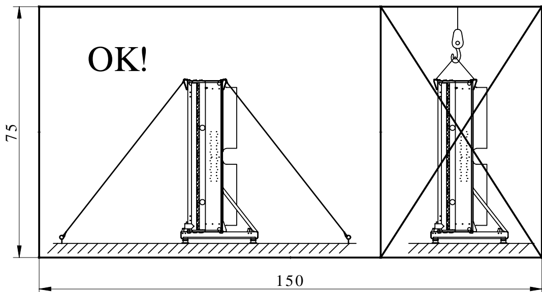
SP 08 szerinti kötőfeszítés
