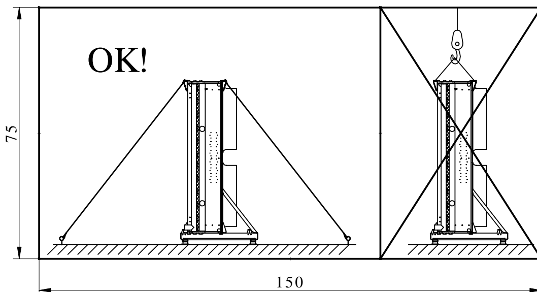
Arriostramiento de cable conforme a SP 08
