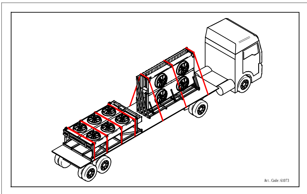
28 - Hinweis Verzurröse für Transport
