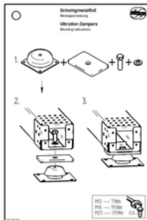
79 - Hinweis "Schwingungsmetallfüße"
