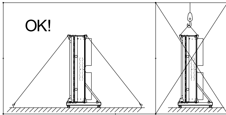
24 – Hinweis auf korrekte Seilverspannung, nur bei vertikaler Bauweise
