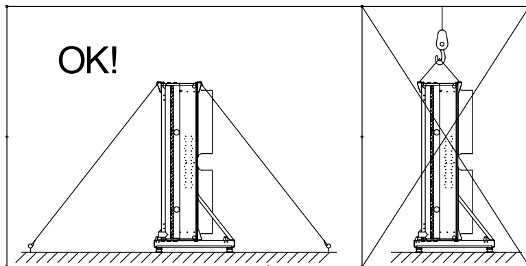
24 – Henviſning til korrekt wire-fastspænding, kun for vertikal konstruktion
