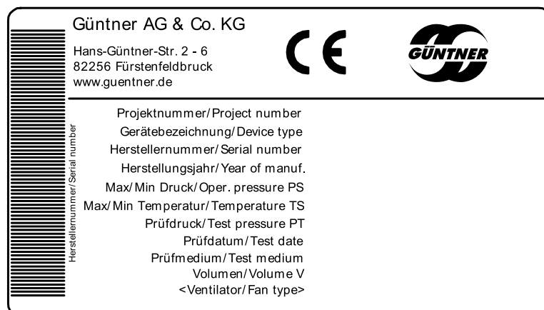
1 - фабрична табелка
