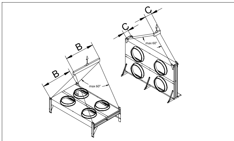
21 - транспортно предписание
