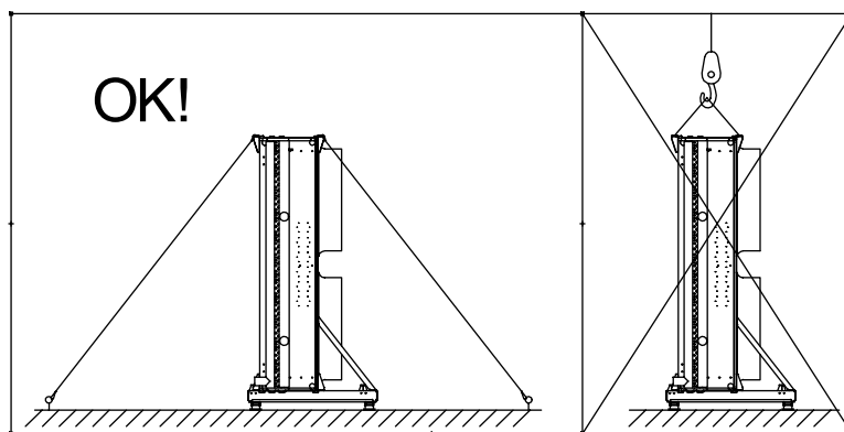
24 - указание за правилно опъване на въжето, само при вертикална конструкция
