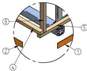
Detaljevisning A
