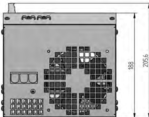
Maße GPHC 580.1
