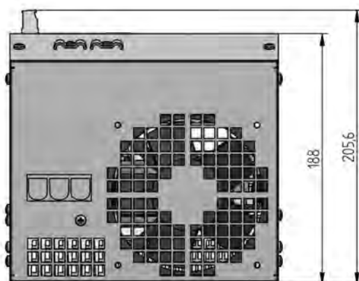
Maße GPHC 380.1
