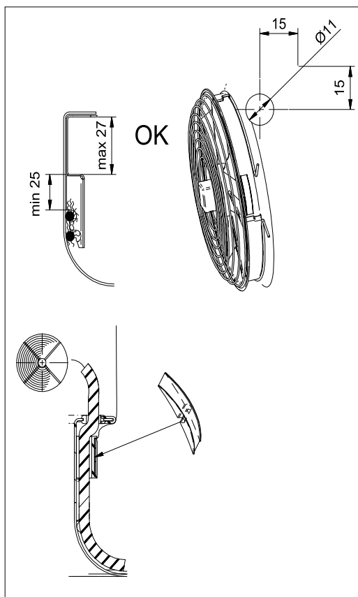
21 - Etiqueta colgante conexión para manga textil (solo en caso de conexión para manga textil opcional) Solo en GHN 071.2 - 080.2 con conexión para manga textil opcional
