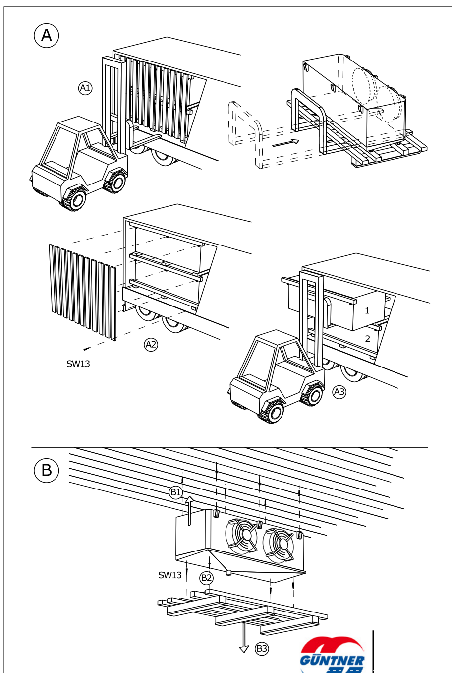
15 - използване на вилков електрокар (видно на опаковката)
