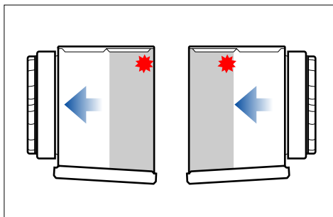
Препоръчително разполагане на датчика за размразяване
