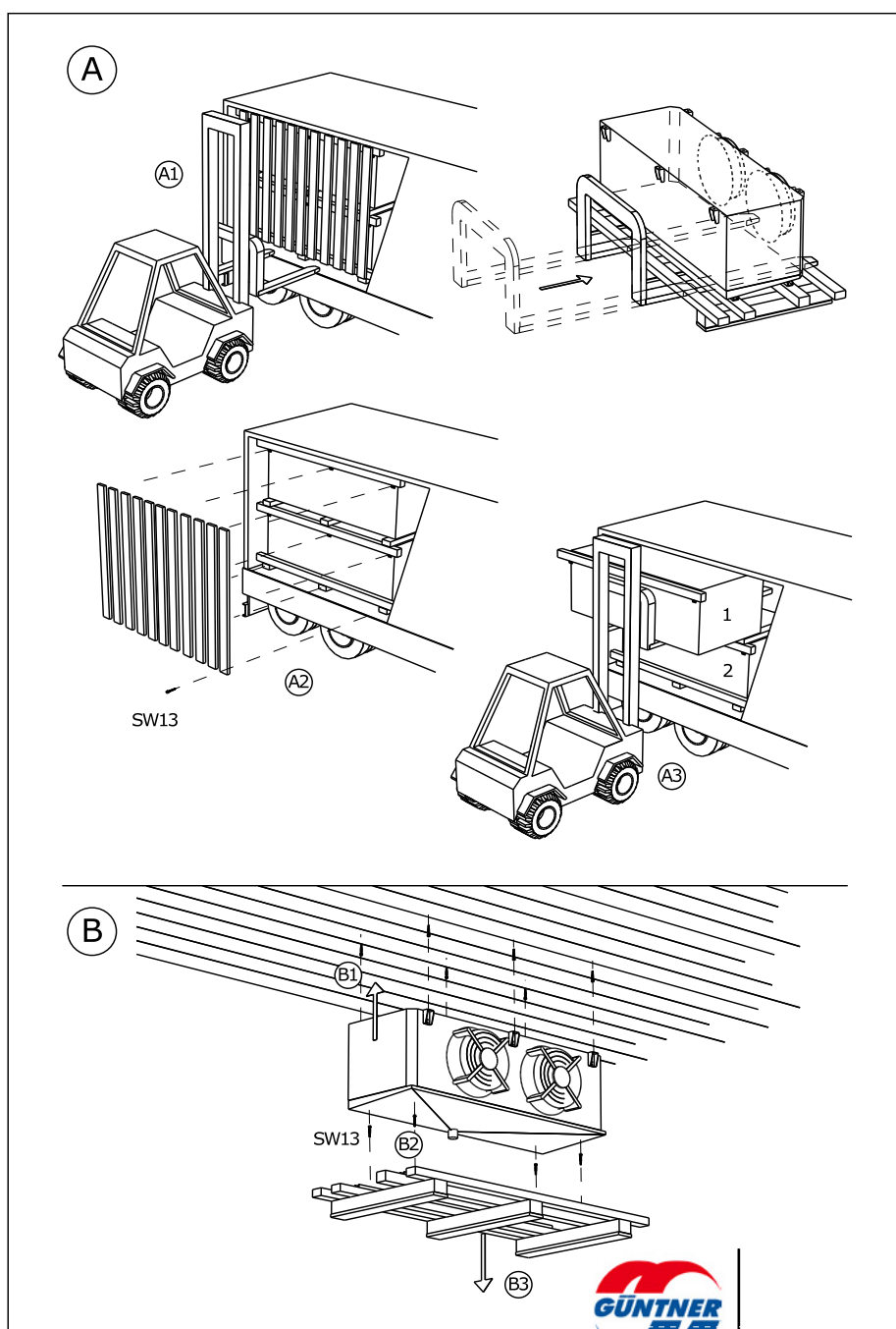
15 - Staplereinsatz (sichtbar auf Verpackung)
