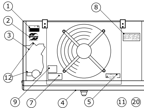
Platzierung von Kennzeichnungen am Gerät
