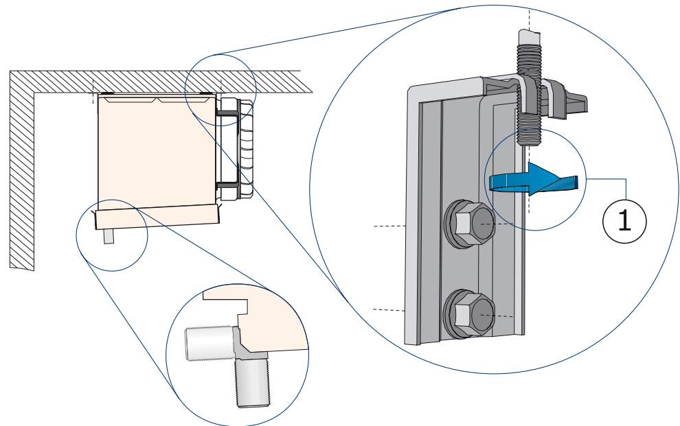
Deckenbefestigung (serienmäßig an den Aufhängern)
