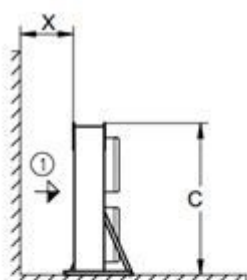
Installazione libera
