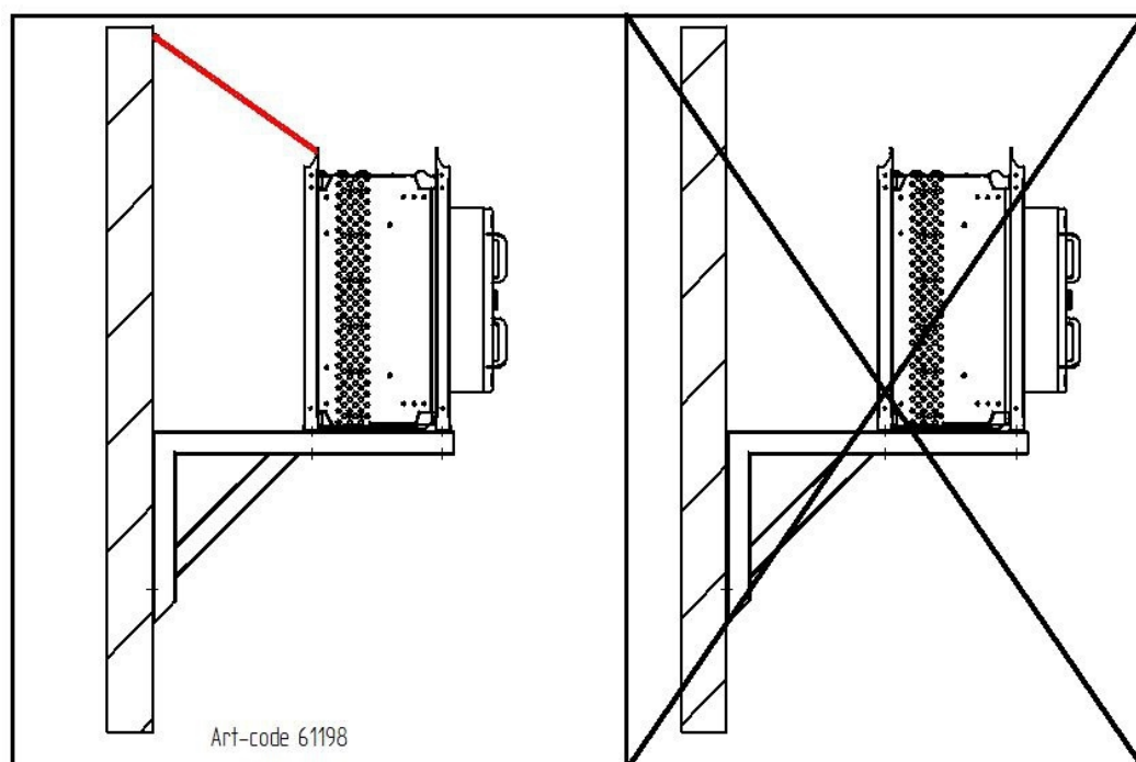
61198 - Indicazione ancoraggio per console a parete
