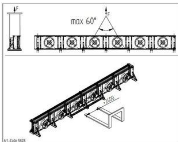
5828 - Uso di gru o carrello elevatore per apparecchi di tipo II + III
