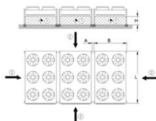
Installazione composta
