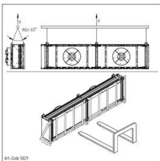
5829 - Uso di gru o carrello elevatore per apparecchi di tipo I
