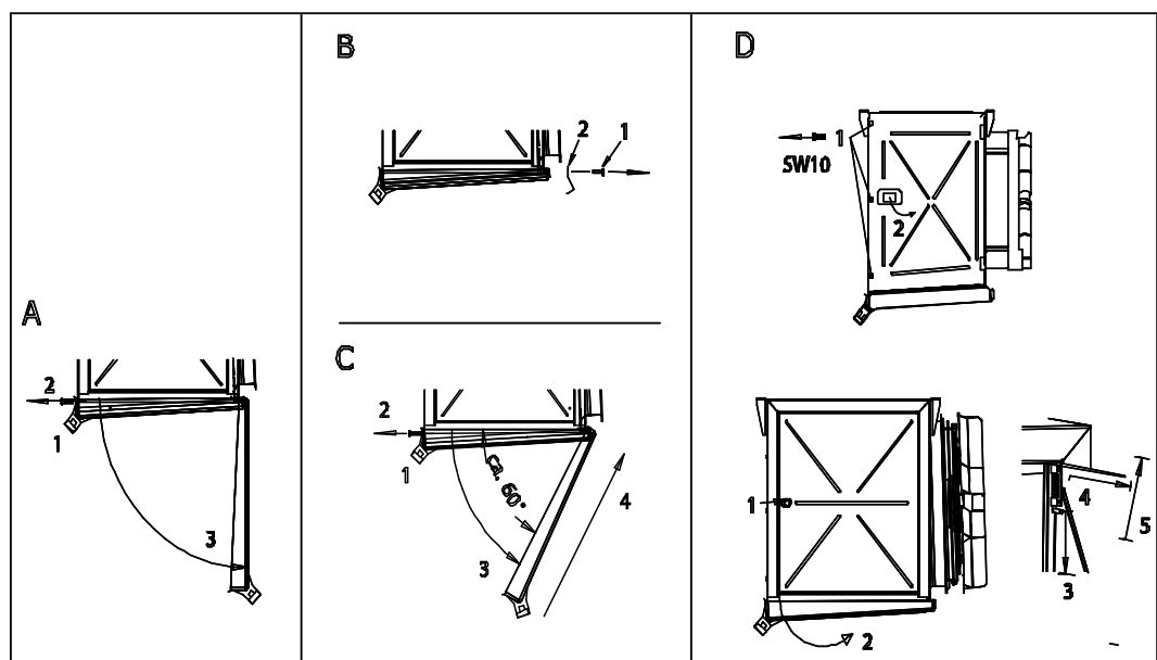
Tropfwanne und Seitenverkleidung demontieren
