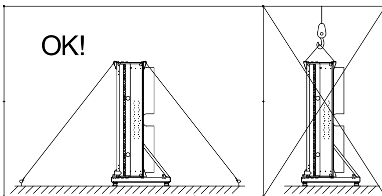
24 – Upozornění na správné napnutí lana, jen při svislé montáži
