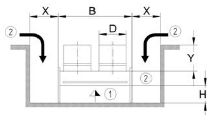
Instalace v šachtě budovy - výfukové trysky
