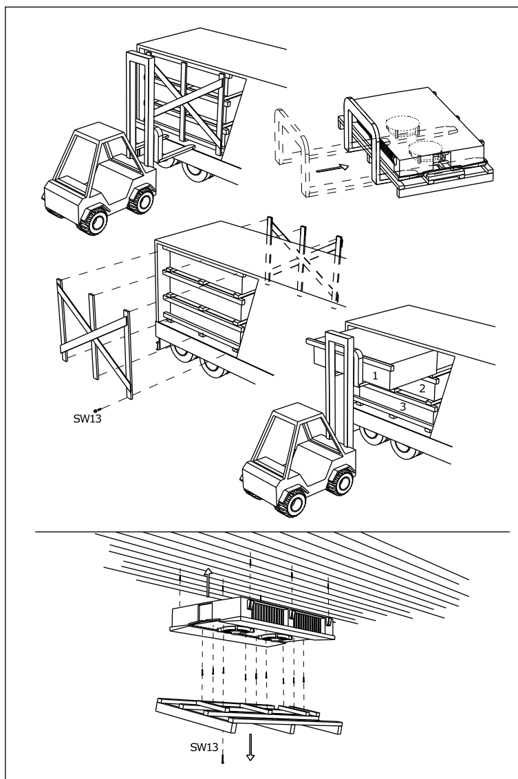
20 - Прицеп, монтаж потолочного воздухоохладителя
