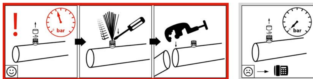
940 - Avviso "Riempimento di trasporto" sulla valvola Schrader
