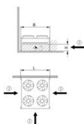
Installazione sulla parete di un edificio
