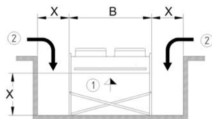
Installazione nel pozzetto di un edificio
