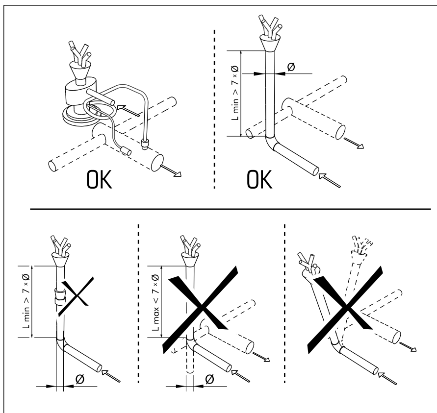
13 - Montáž expanzního ventilu
