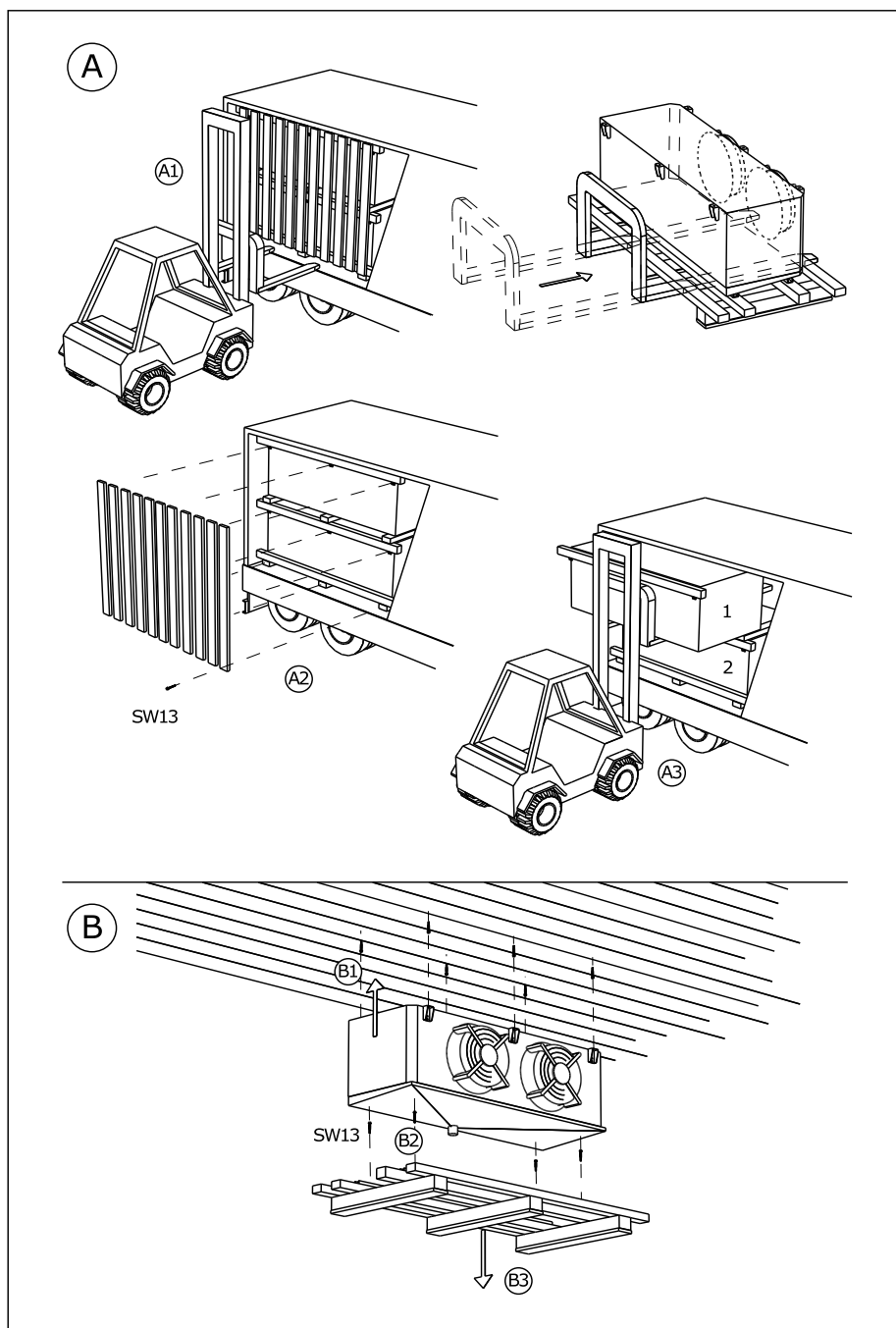
17 - Závěsný štítek Montáž vzduchového chladiče pod strop
