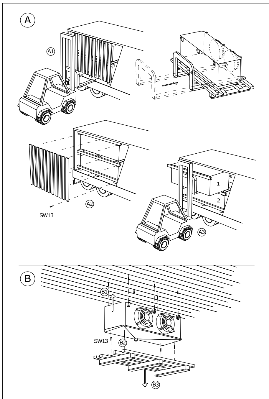
17 - маркиращ етикет монтаж таванен въздушен охладител
