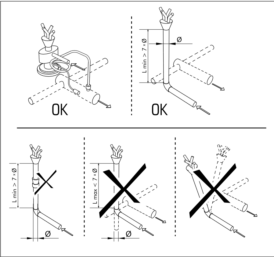
13 - монтаж терморегулирующ вентил
