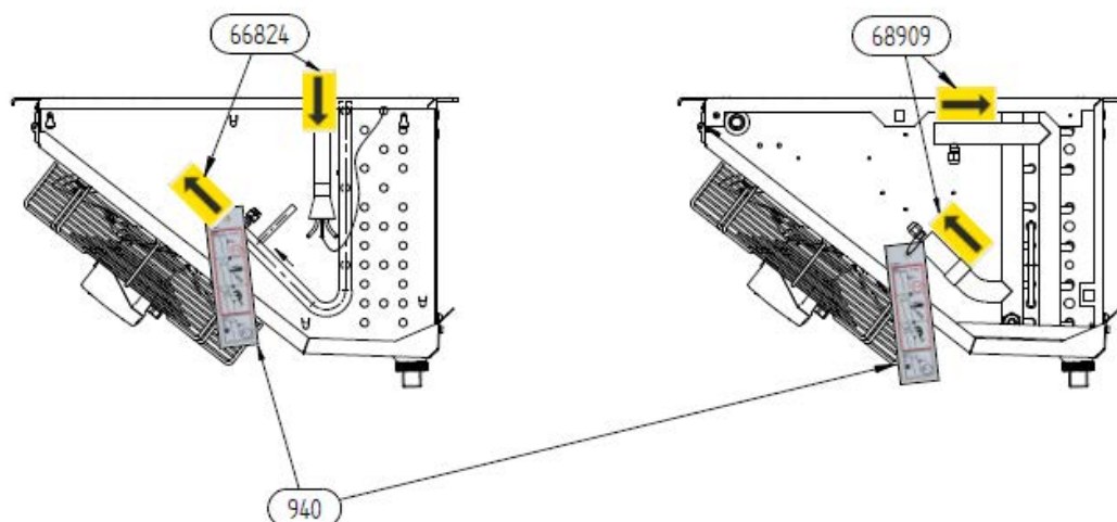
A GASC RX, ill. CX (balra) és a GASC FP (jobbra) csatlakozási oldala
