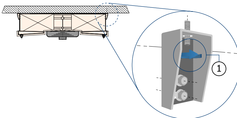
Закрепване на тавана (серијно на приспособленията за окачване).
