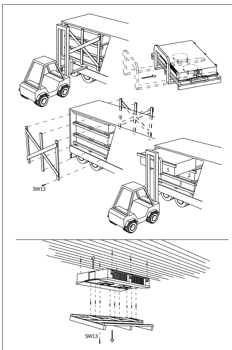
15, 17, 26 - монтаж таванен въздушен охладител
