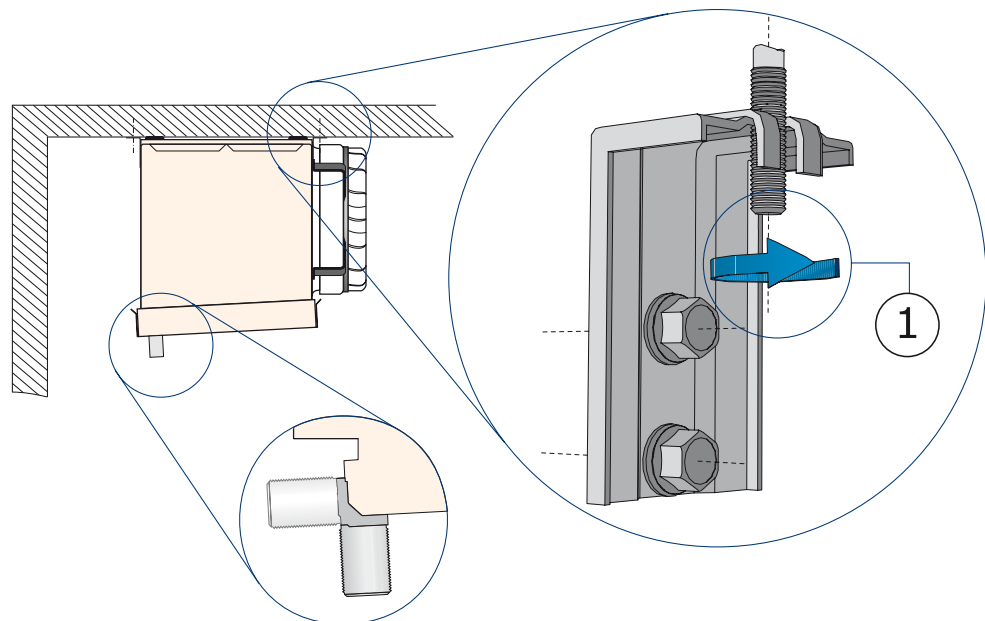
Fissaggio a soffitto (di serie sugli agganci)
