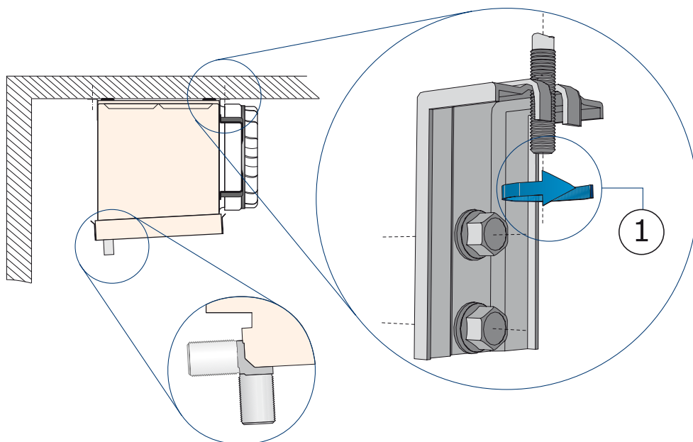
fixation plafonnrière (de série à des attaches)
