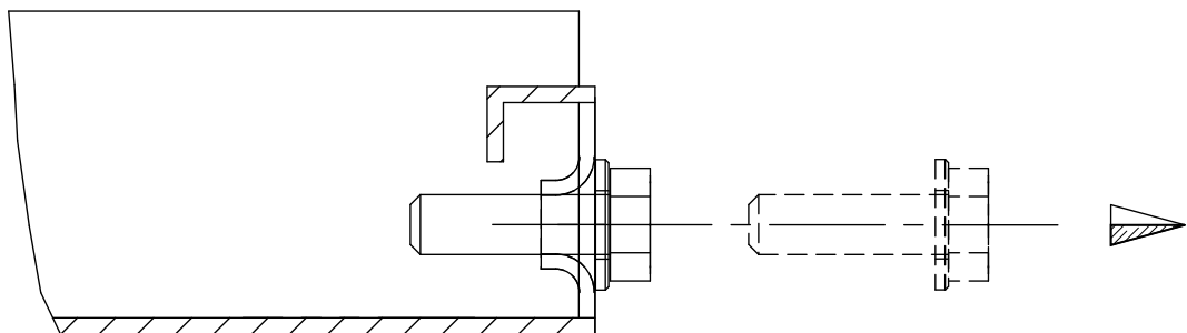
Desserrage de la vis pour le démontage du bac de la série DHF
