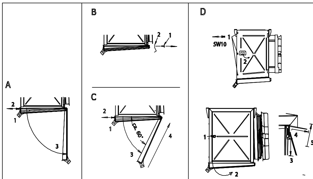
Demontera spillträget och sidobeklädnaden
