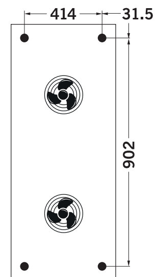
GAMC 020.1/2**/DX***
