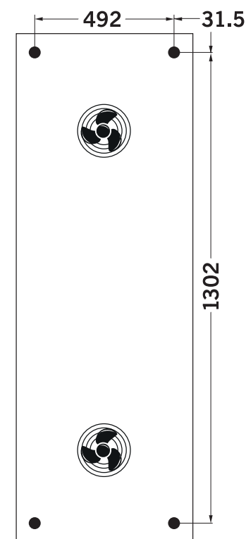
GAMC 020.1/2**/HY***
