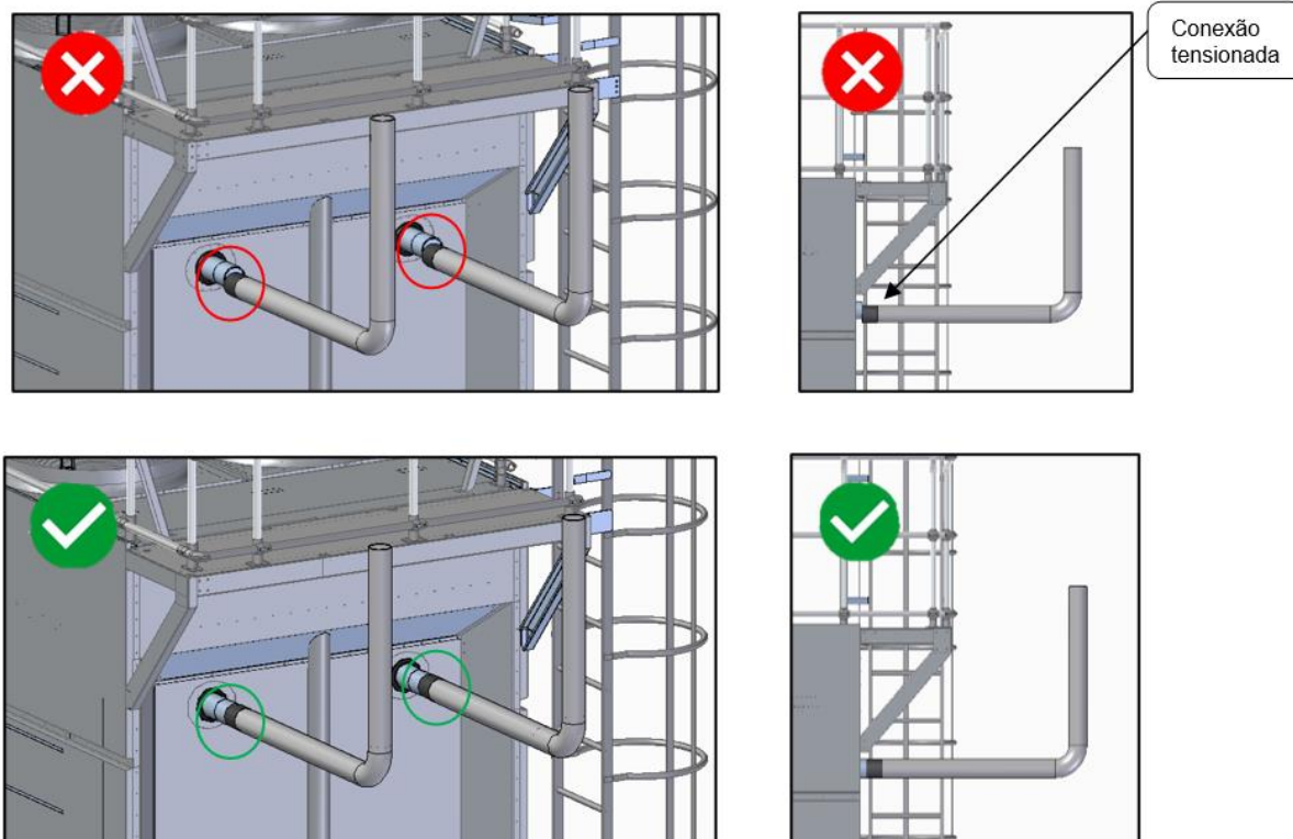
Figura 1 – Instalação de tubulações
