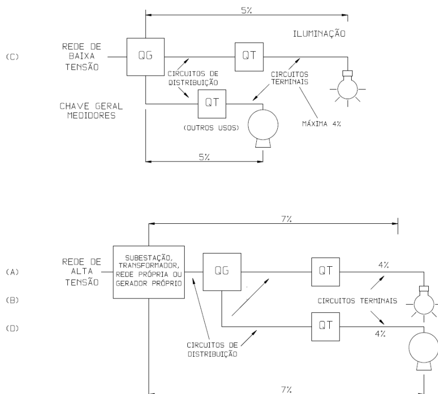
Figura 1 - Esquemático Limites de Queda de Tensão da NBR 5410:2004
