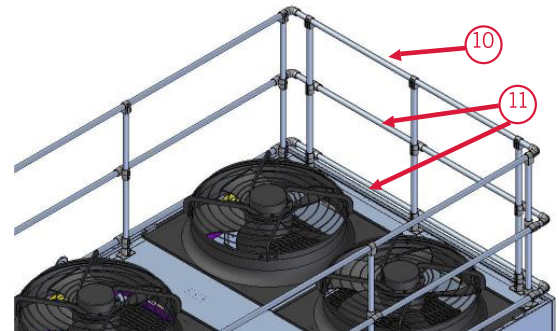
Figura 9: Tubos traseiros do guarda corpo.
