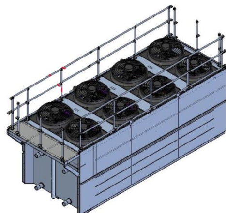
Figura 8: Tubos laterais do guarda corpo.
