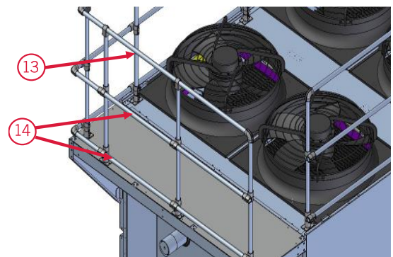
Figura 12: Tubos frontais do guarda
