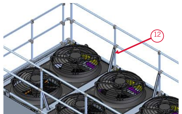
Figura 11: Reforços do guarda corpo.
