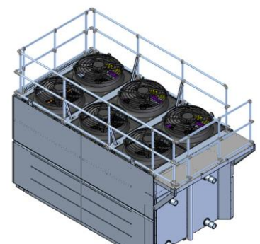
Figura 13: Montagem final.
