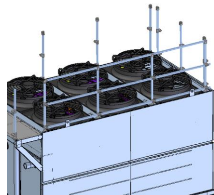
Figura 6: Tubos laterais do guarda corpo.
