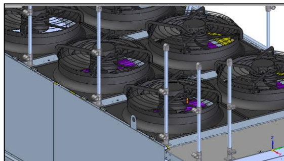
Figura 3: Montagem das colunas do guarda corpo.
